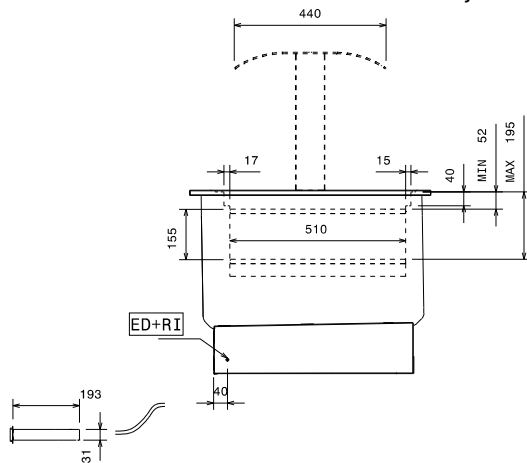
Zij aanzicht
